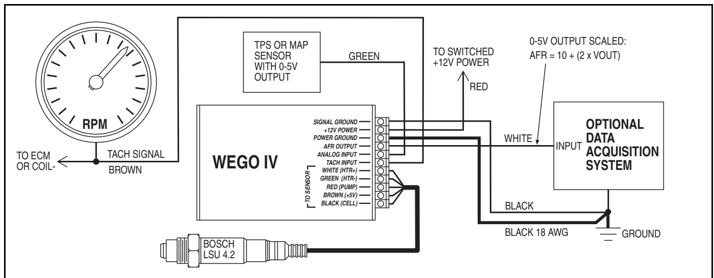
Figure 1 - WEGO IV Hookup
