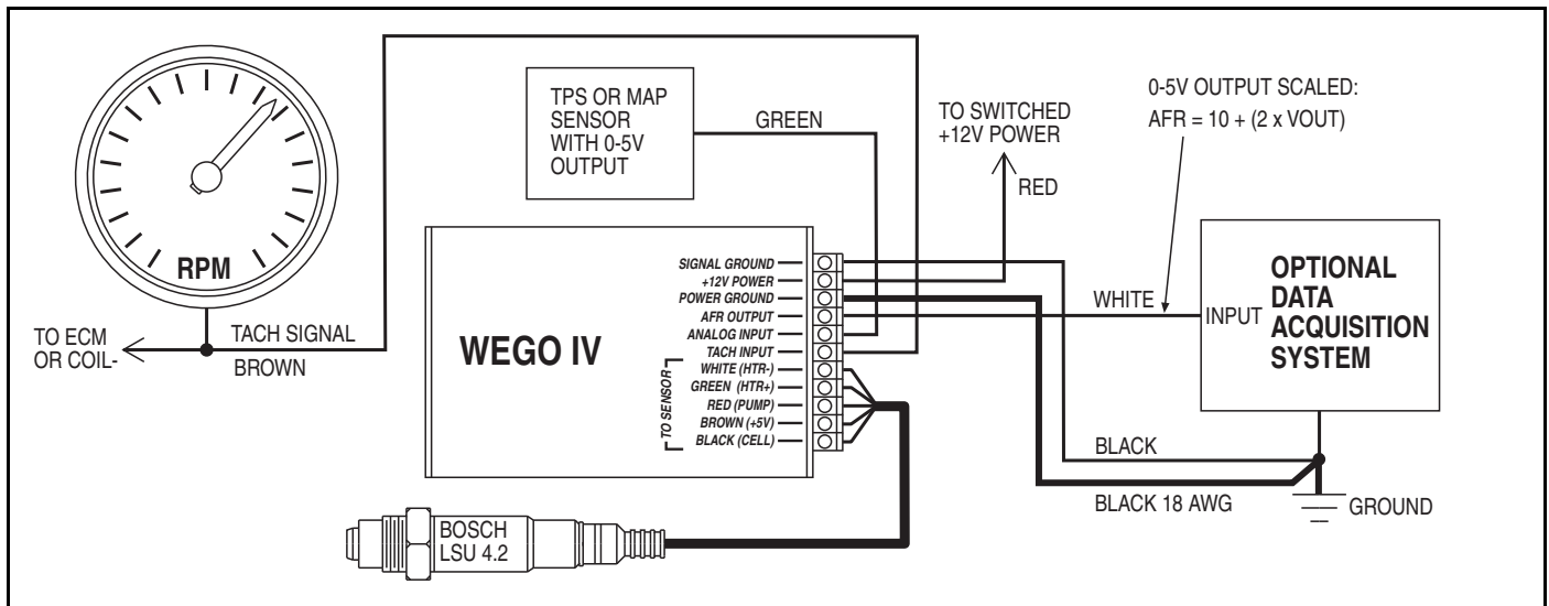
Figure 1 - WEGO IV Hookup
